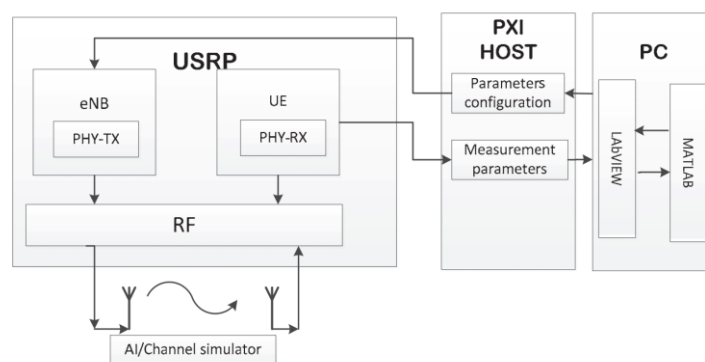
Figura 1. Plataforma LTE de hardware en el lazo de simulación
